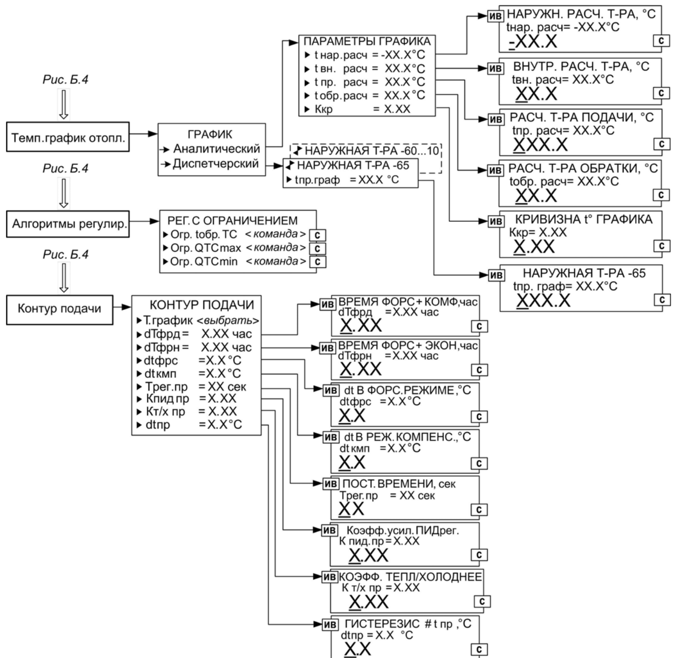
Рис.Б.5. Подменю Температурный график отопления, Алгоритмы регулирования и Контур подачи
