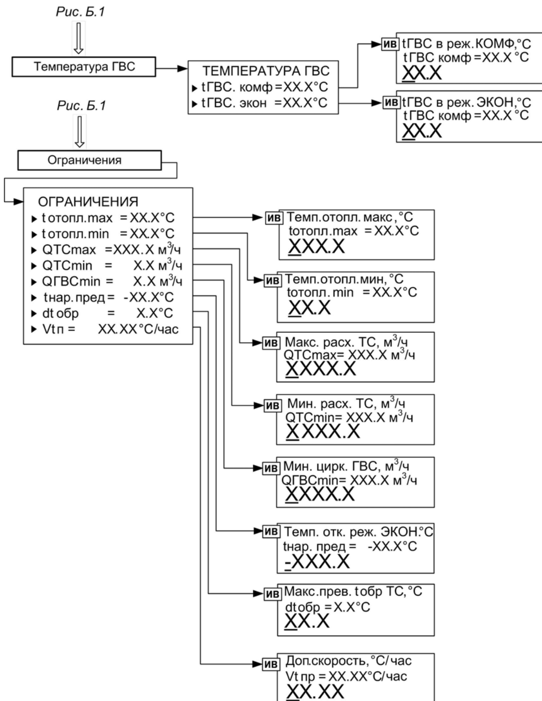
Рис.Б.2. Меню Температура ГВС и Ограничения
