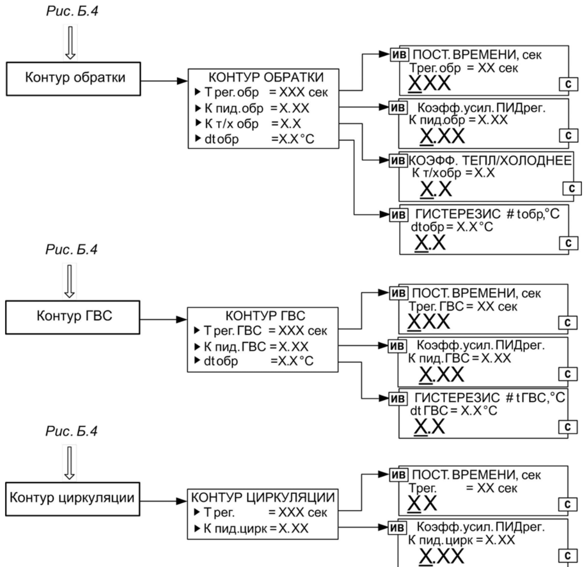
Рис.Б.6. Подменю Контур обратной, Контур ГВС и Контур циркуляции
